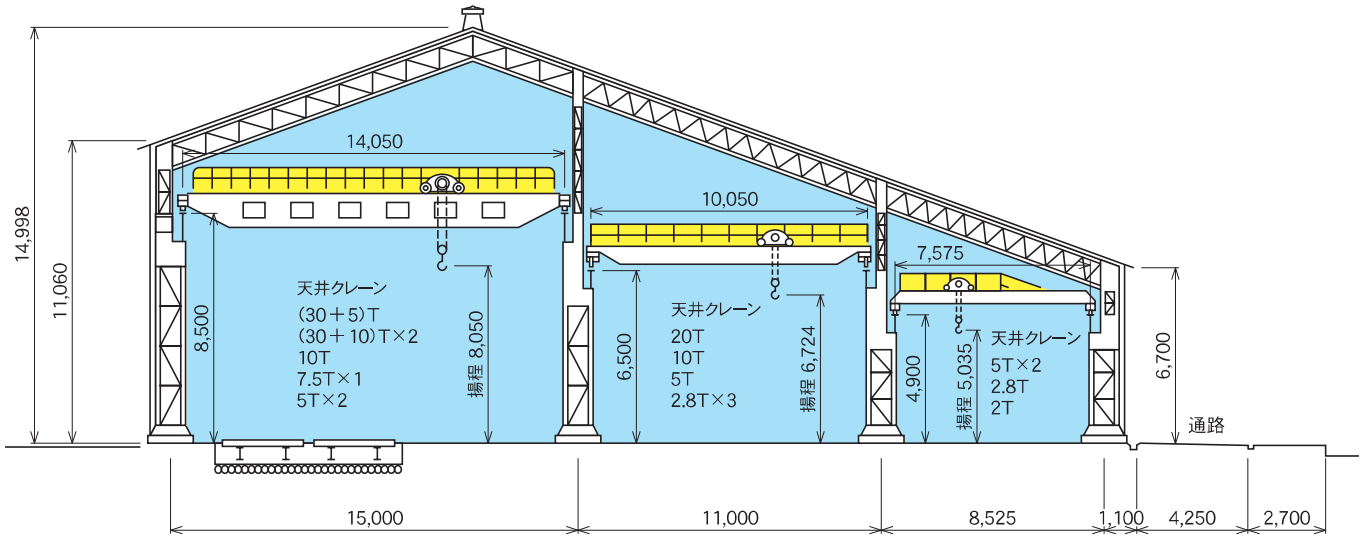
① 第一工場
